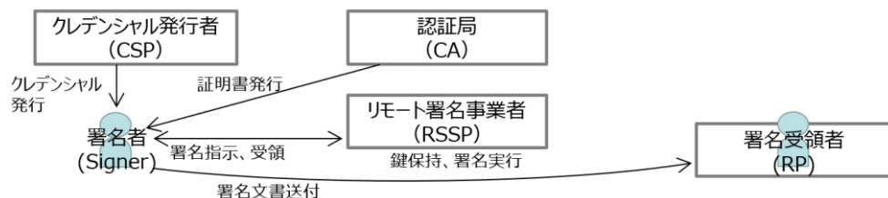
図 3-3 ローカル署名モデルとリモート署名モデルの比較（プレイヤーと保有情報）
