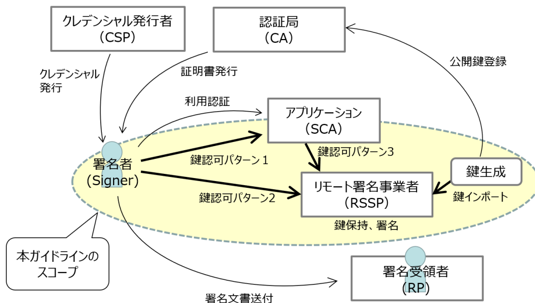
図 3-5 リモート署名における本ガイドラインのスコープ
