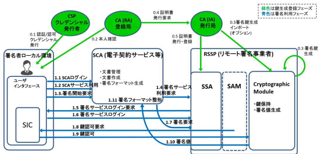
図 5-2 基本モデル1 (SCAからのリモート署名サービス利用)
