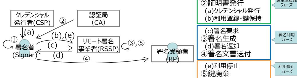
図 4-5 ローカル署名モデルとリモート署名モデルの比較（処理フロー）
